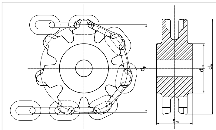
Ruota alveolata - Pocket wheel - Rueda alveolata
