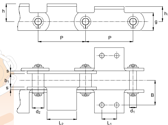
Elevatori a tazze Bucket elevators Elevadores de cangilones
