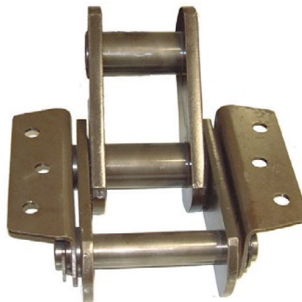
Esempi di tipi per le alette di attacco. Examples of types of attachments. Ejemplo de tipos para las aletas de sujeción.
