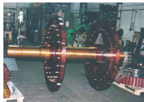
Gruppo motrice Driving group Estación motriz
