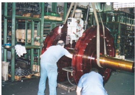
Montaggio gruppo motrice Driving group assembly Montaje estación motriz
